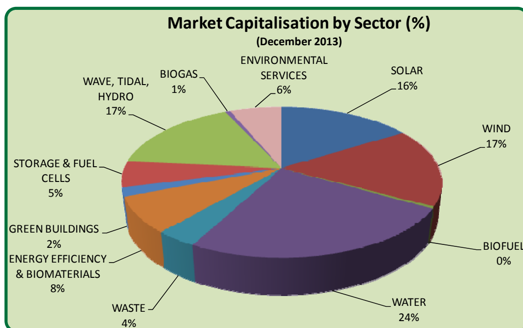
各个行业的总市值 (%) (2013 年 12 月)
